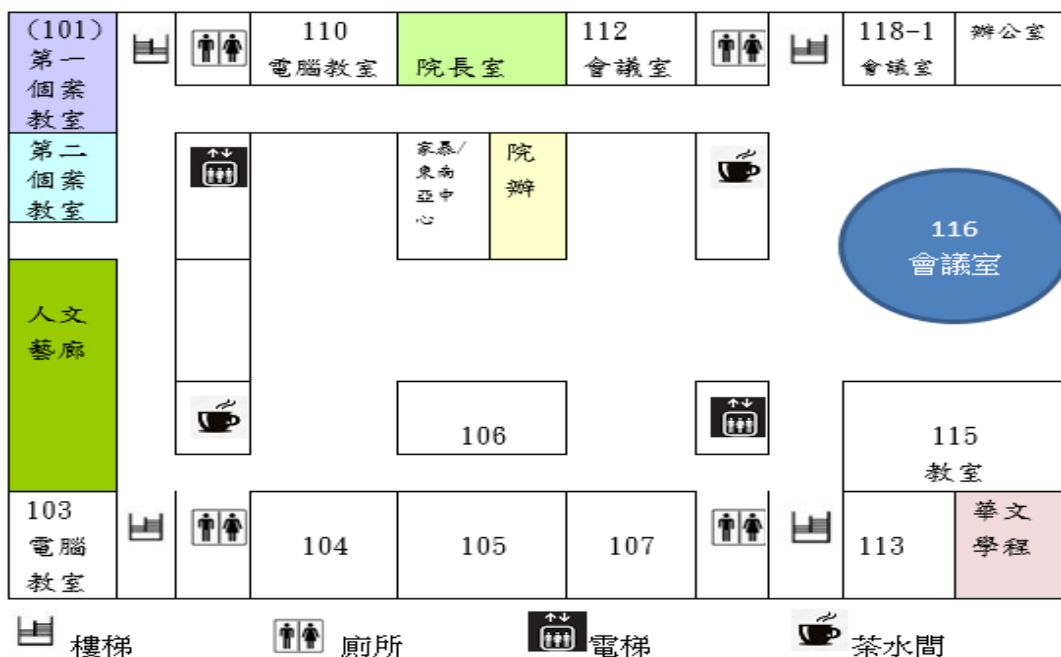
人文學院平面圖---1樓
